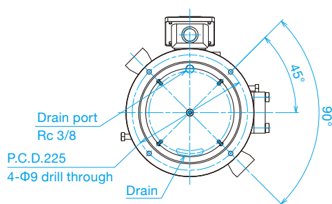
300 L Type
