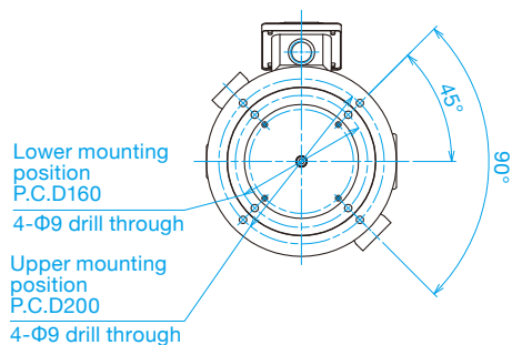
150 L Type
